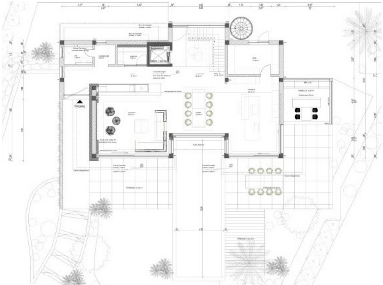
Grundriss EG
