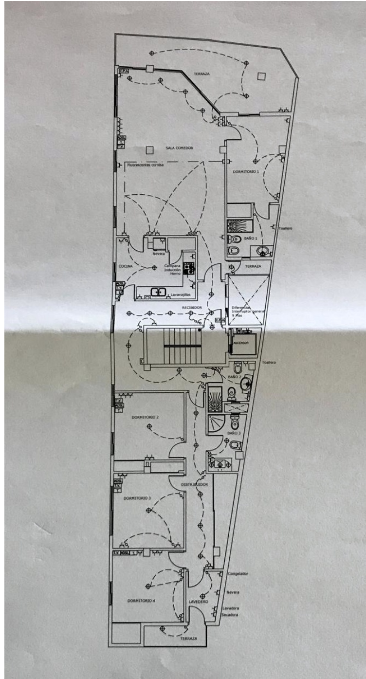
Grundriss
