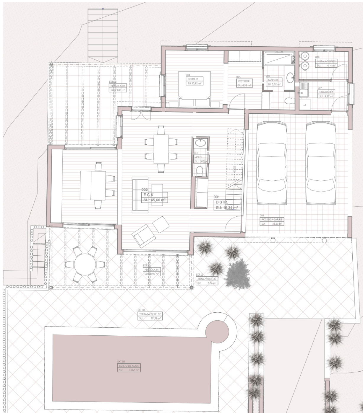
Grundriss Erdgeschoss
