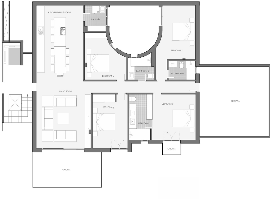
Plano Planta 2
