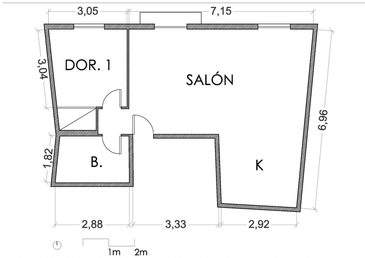
Grundriss
