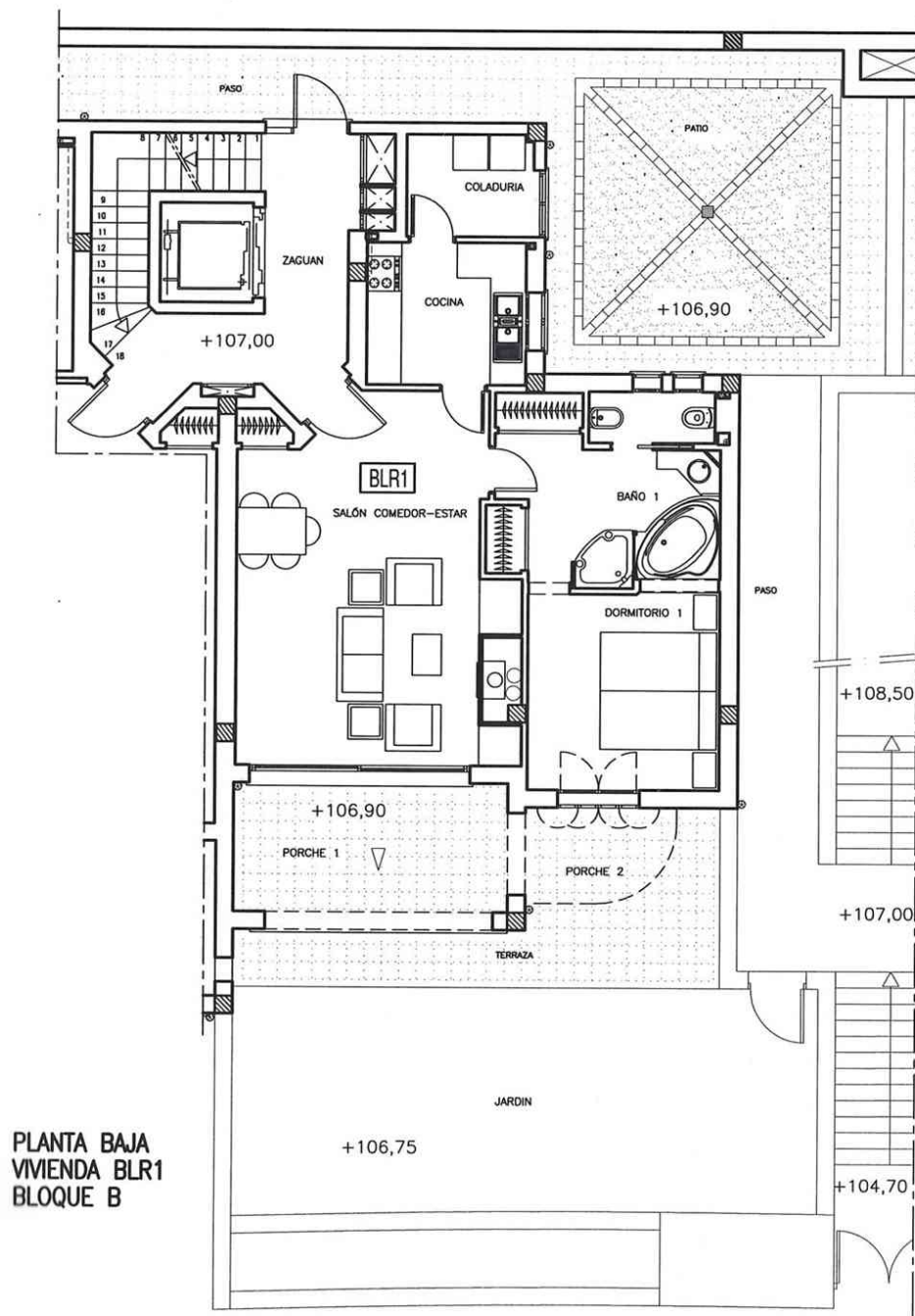
Grundriss
