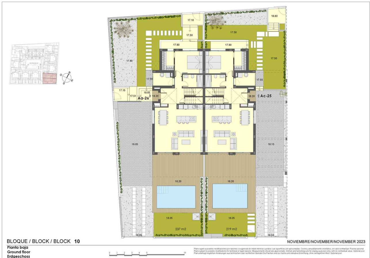
Grundriss Haus 26 (Erdgeschoss)
