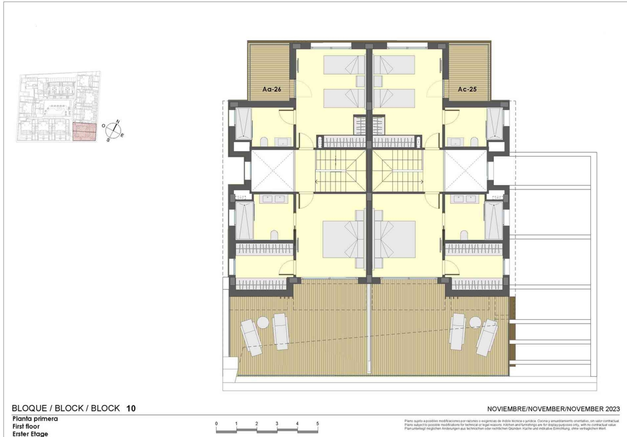
Grundriss Haus 26 (Obergeschoss)
