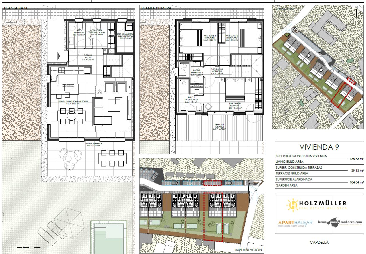
Plano_Vivienda9
