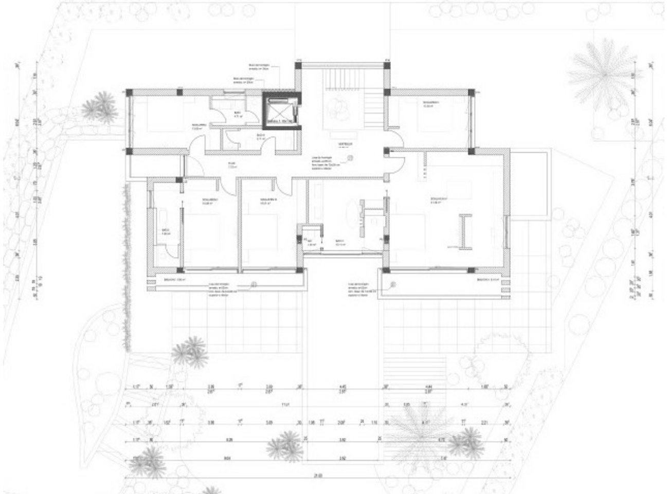
Grundriss OG
