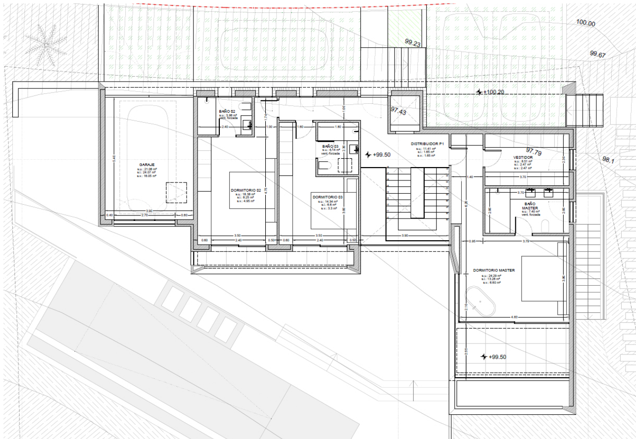
Plano_Planta_Piso
