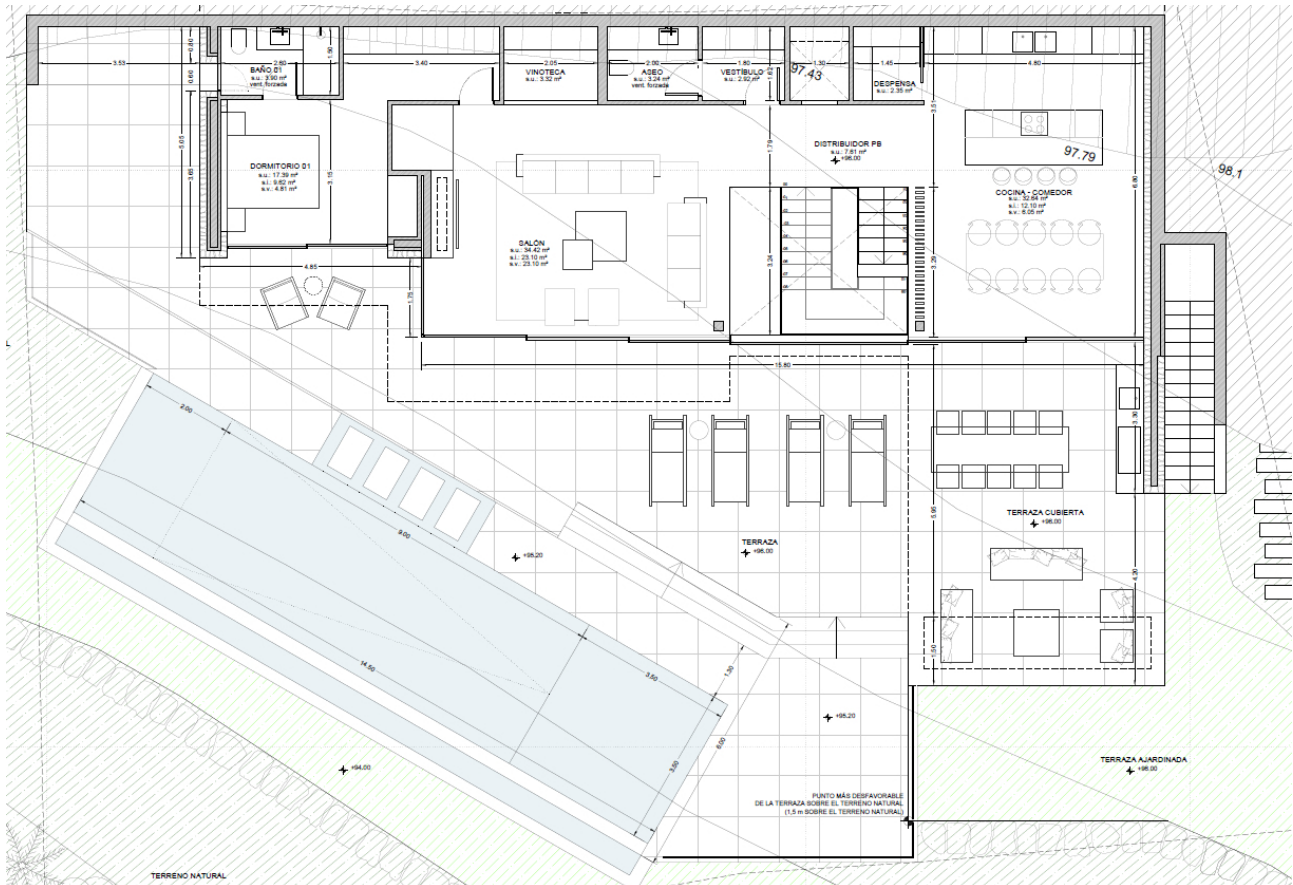
Plano_Planta_Baja
