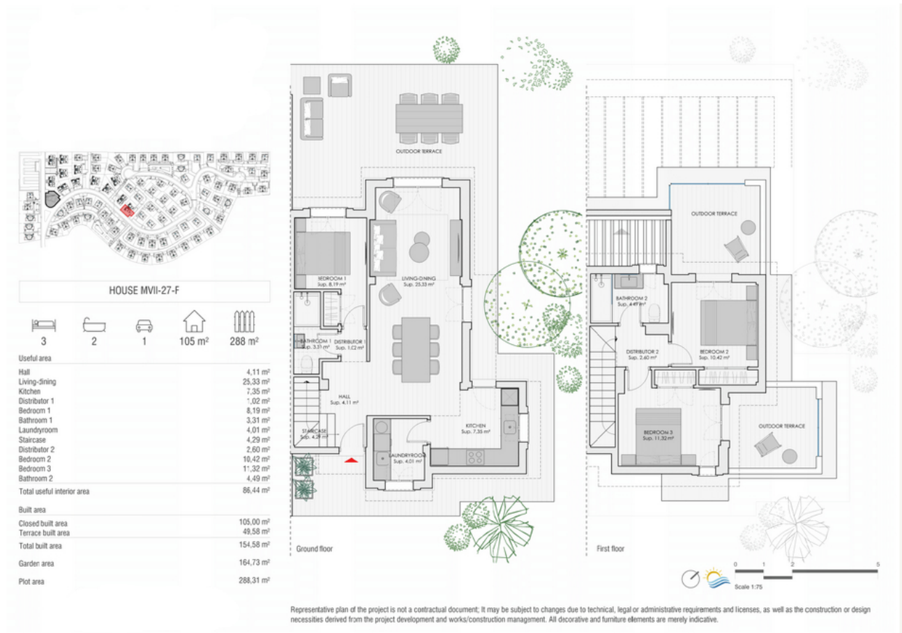
Plano MVII-27-F
