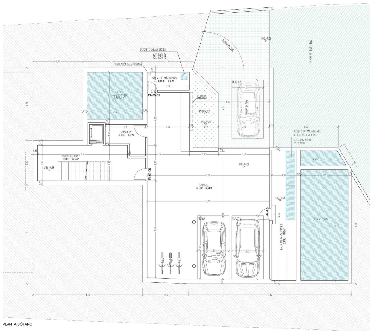
4 Planta arquitectonica del sotano -
