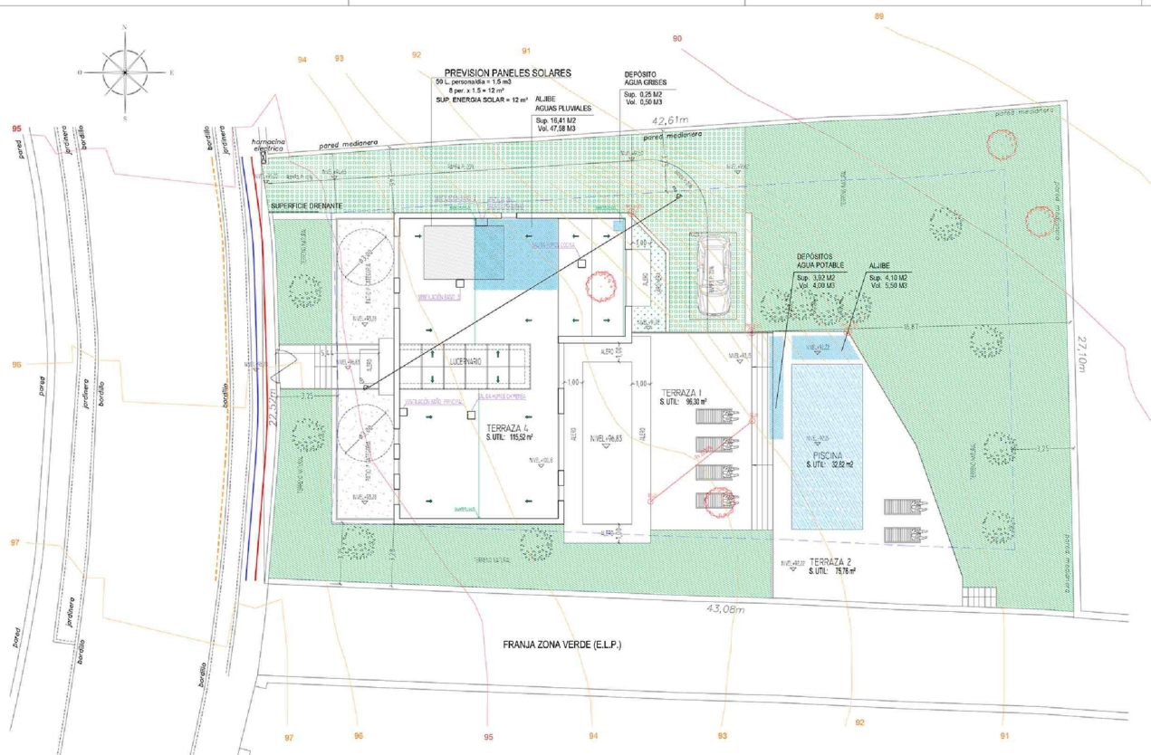
1 Planta arquitectonica general del primer nivel
