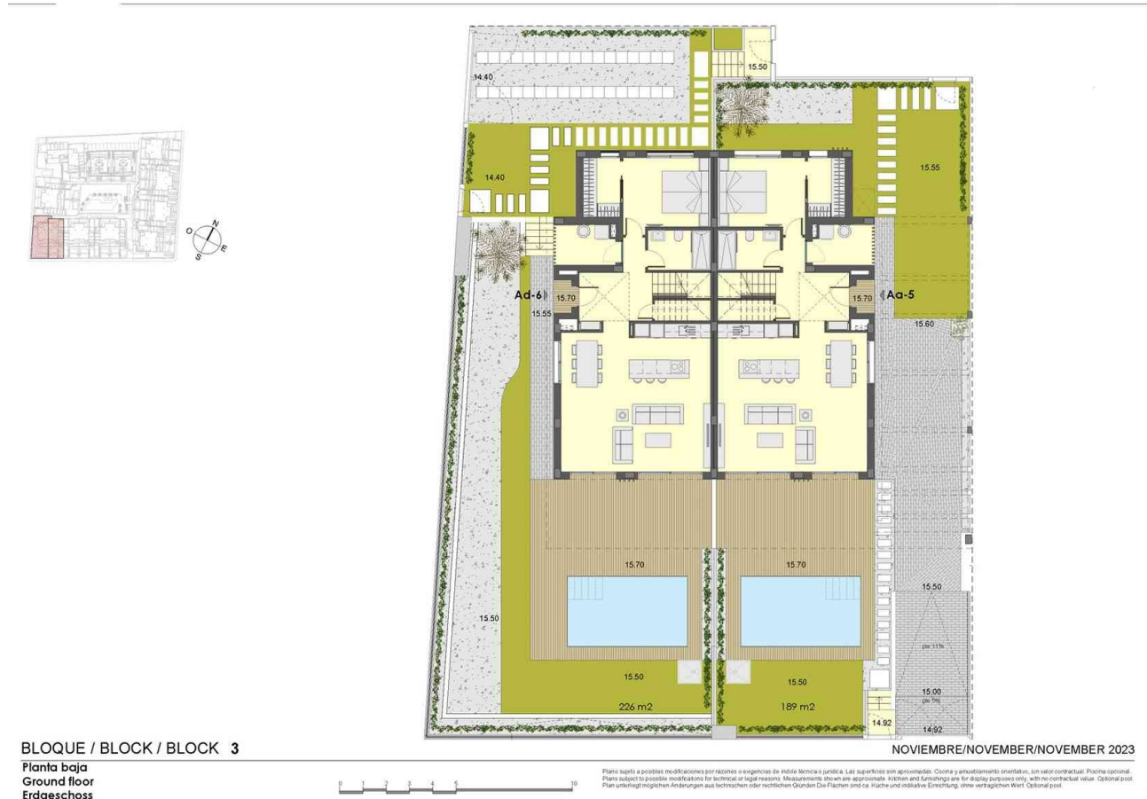
Plano Villa 5 (Planta Baja)
