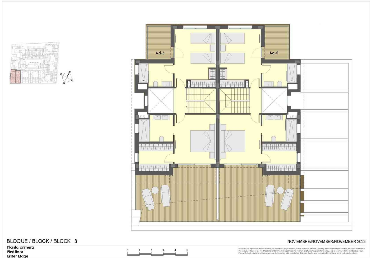
Plano Villa 5 (Planta Piso)
