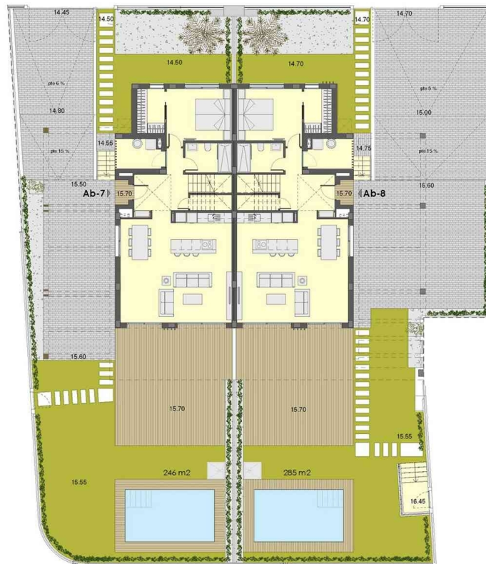
Plano Casa 07 (Planta Baja)
